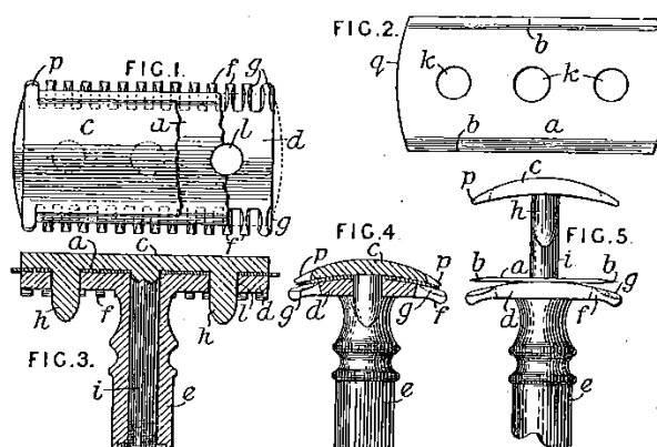
Enkele tekeningen bij het Gillette octrooi uit 1902
