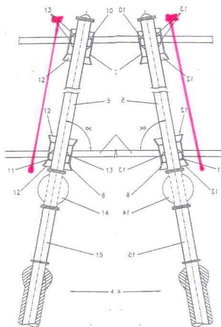
Risers en turret volgens het octrooi
