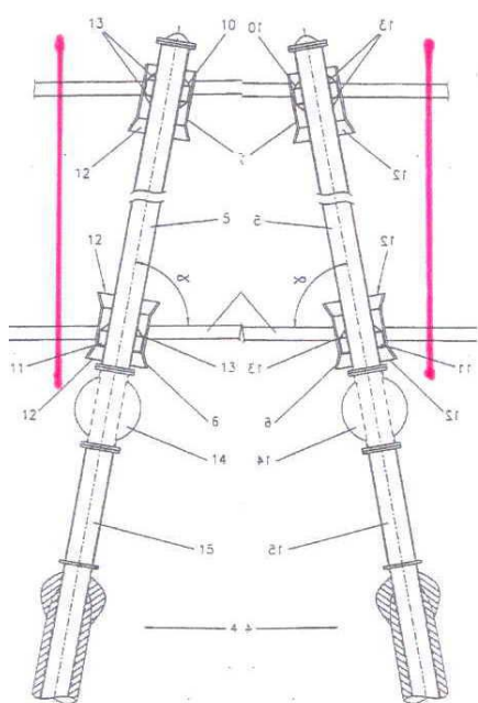
Risers en turret volgens D1
